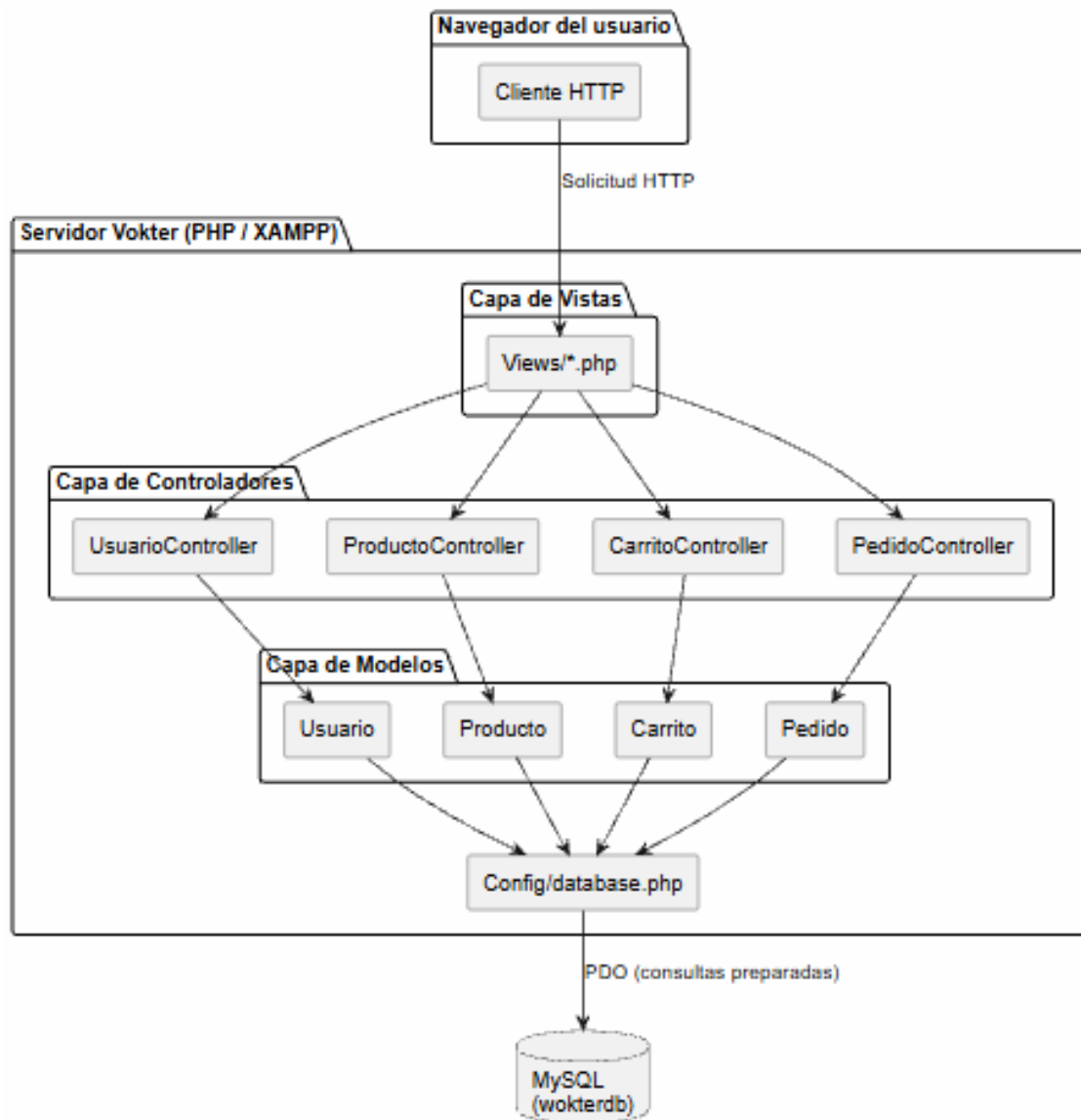
Figura 1. Modelo de capas MVC.
